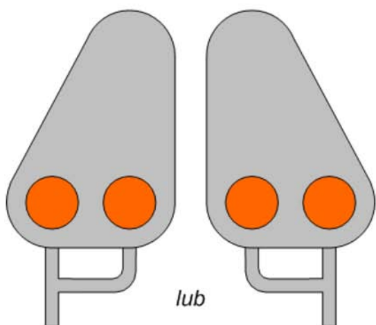
Rys. 45. Sygnał Osp 1
